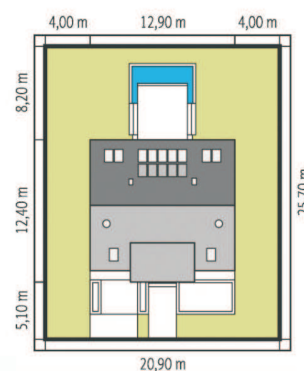
Dimensiuni minime la TEREN
