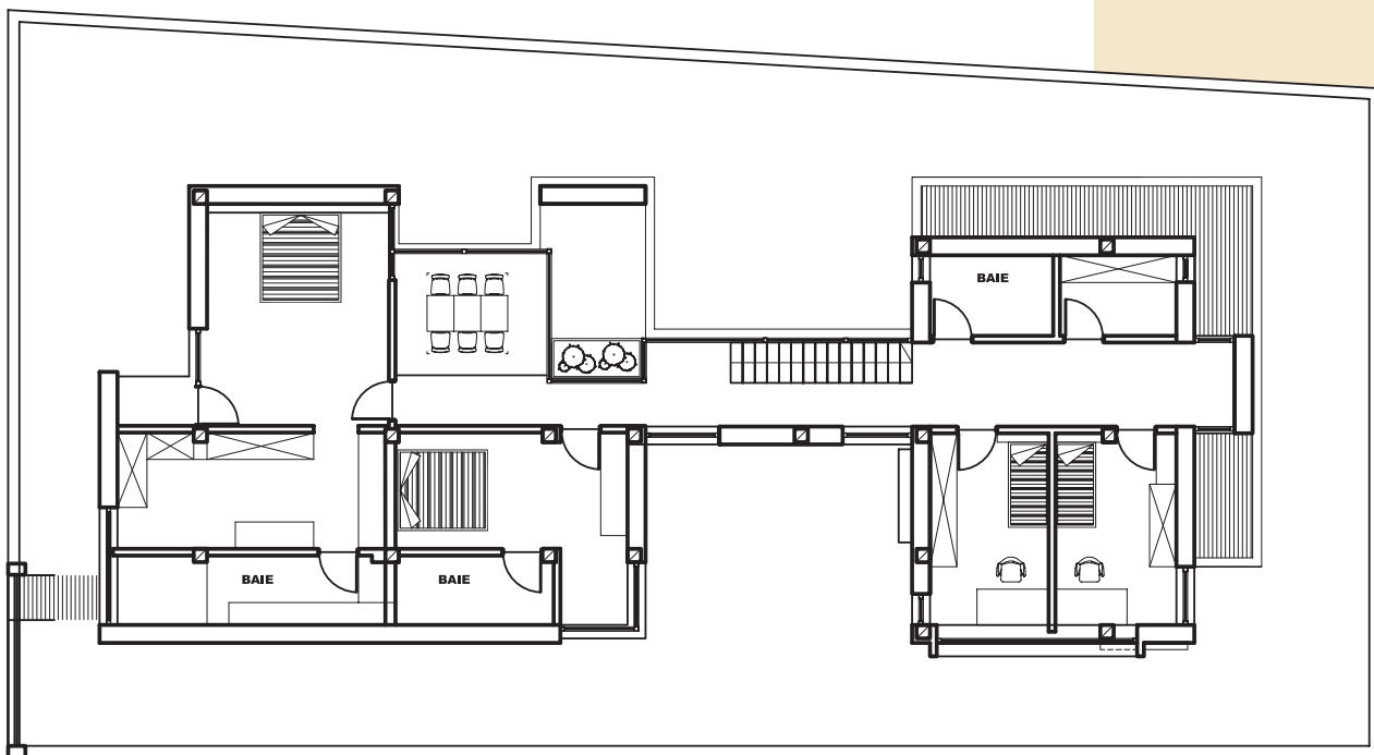
PLAN ETAJ
